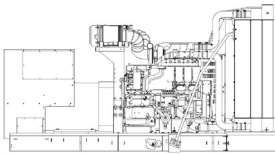
E x B x Y (mm) 1600 x 4500 x 1900 5500 kg.
