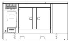
E x B x Y (mm) 1400 x 4000 x 2200 3400 kg.
