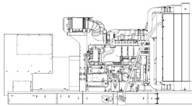
E x B x Y (mm) 1400 x 4000 x 1500 2800 kg.
