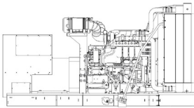
E x B x Y (mm) 1600 x 4000 x 1800 3600 kg.
